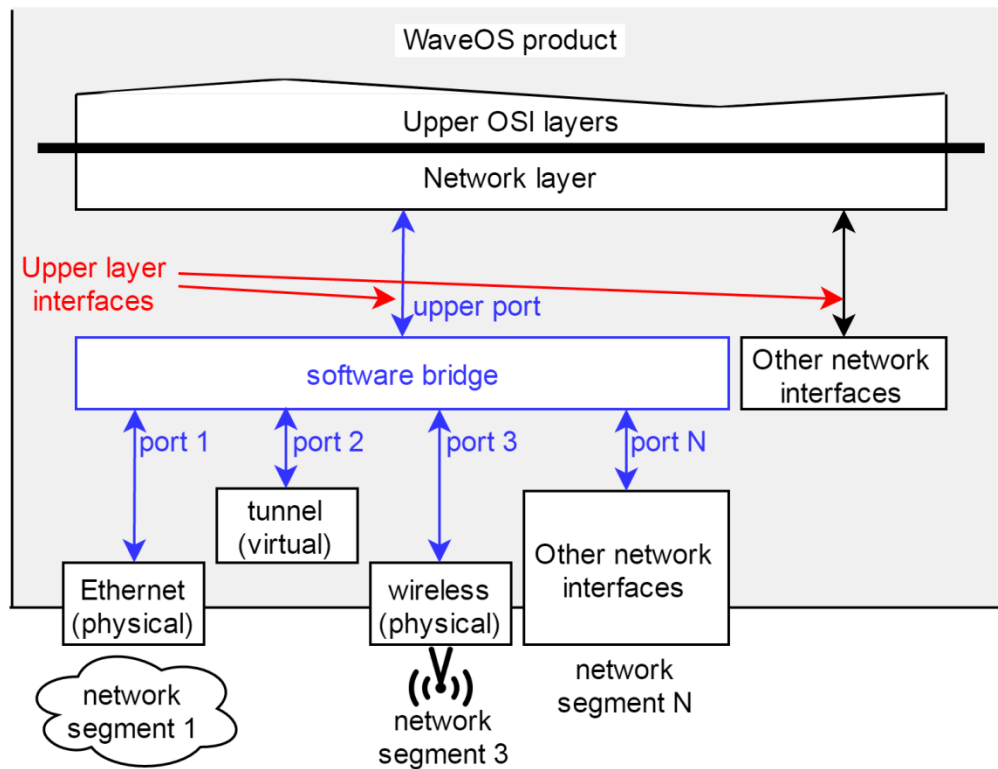
Picture V-5: 소프트웨어 브리지의 상위 계층 인터페이스
