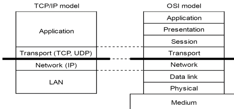
Picture V-2: TCP/IP 모델과 OSI 모델의 비교
