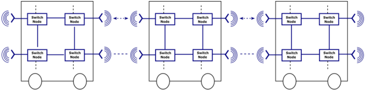
Picture V-9: SRCC 로 구성된 이중화 이더넷 백본의 예시
