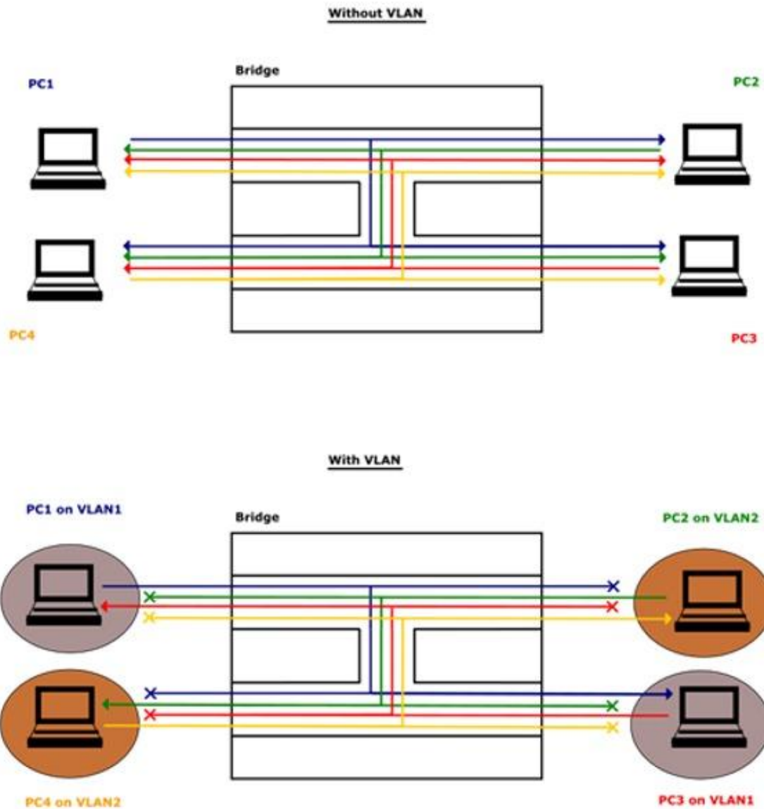
Picture V-3: 컴퓨터는 동일한 VLAN 에 있는 컴퓨터에서만 수신합니다.
