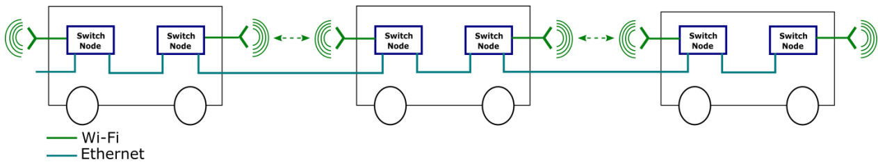
Picture V-10: SRCC 이중화 혼합 모드
